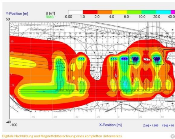
Digitale Nachbildung und Magnetfeldberechnung eines kompletten Unterwerkes Sys tron EMV GmbH
